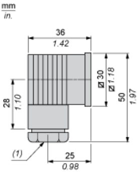
(1) Prensaestopas Pg 11
